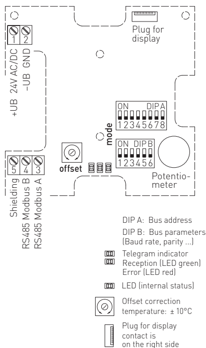
Схема подключения
